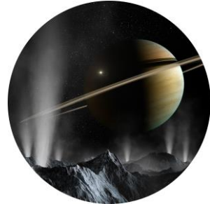
土星の衛星「エンセラダス」の 間欠泉
